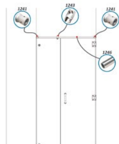
INSTALACION DE MURO A MURO
