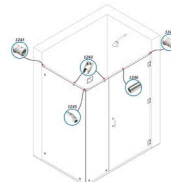
INSTALACION A DE MURO A MURO EN ANGULOS INDISTINTOS (EJEMPLO A 135°)
