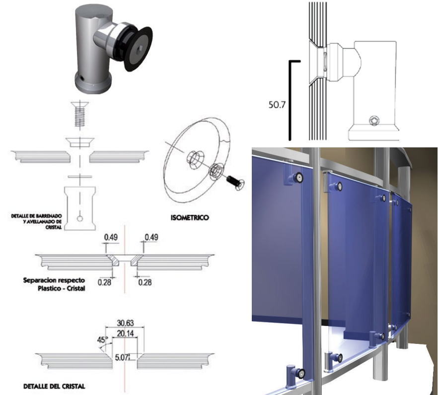
CONECTOR MORELOS MURO-VIDRIO P/VIDRIO DE 8 A 12MM
