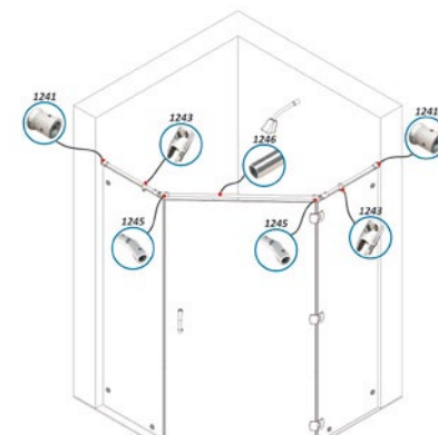
INSTALACION A DE MURO A MURO EN ANGULOS INDISTINTOS (EJEMPLO A 135°)
